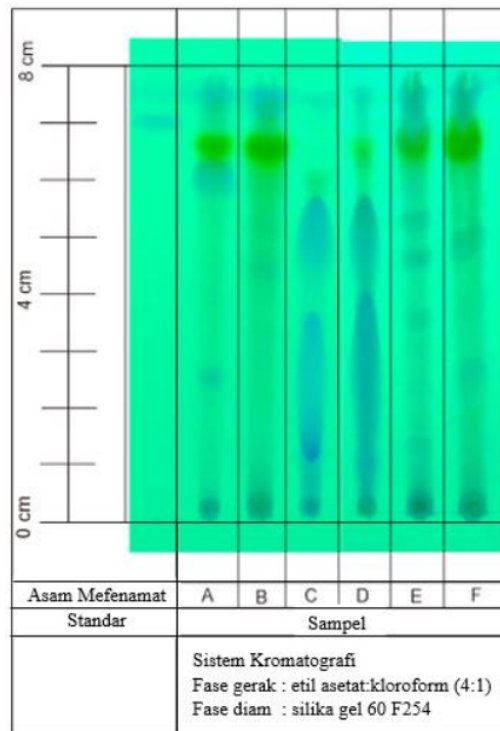
Gambar 2. Kromatogram Hasil Elusi Sampel dan Standar Asam Mefenamat
