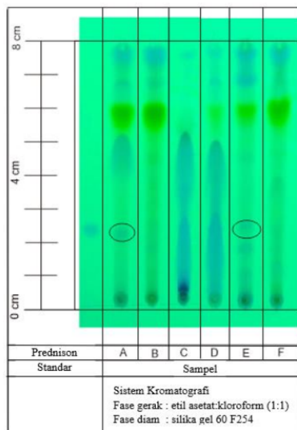
Gambar 3. Kromatogram Hasil Elusi Sampel dan Standar Prednison
