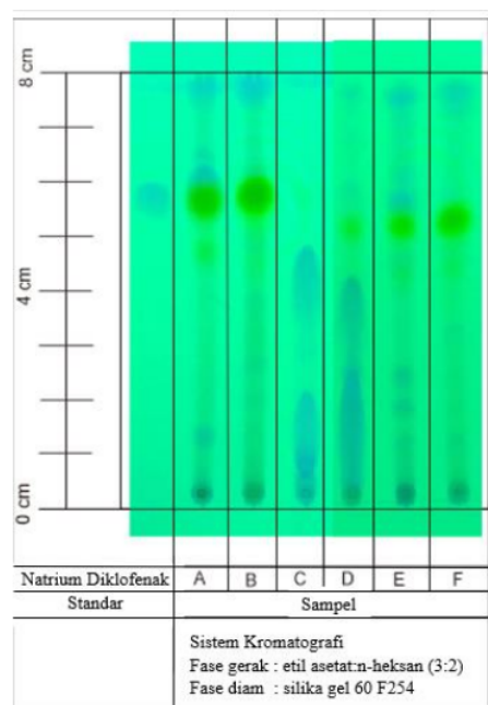
Gambar 4. Kromatogram Hasil Elusi Sampel dan Standar Natrium Diklofenak
