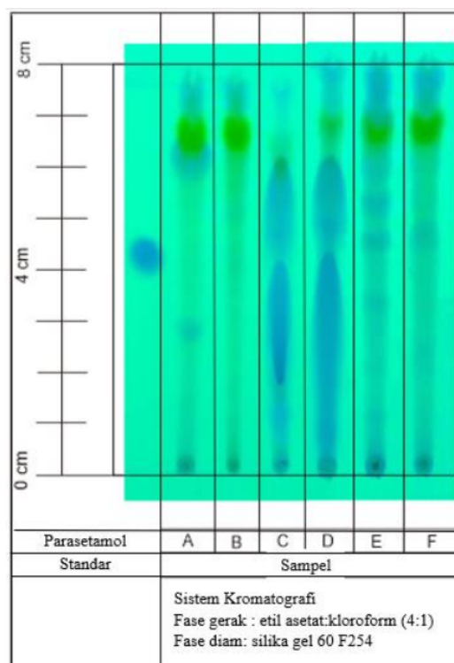
Gambar 1. Kromatogram Hasil Elusi Sampel dan Standar Parasetamol
